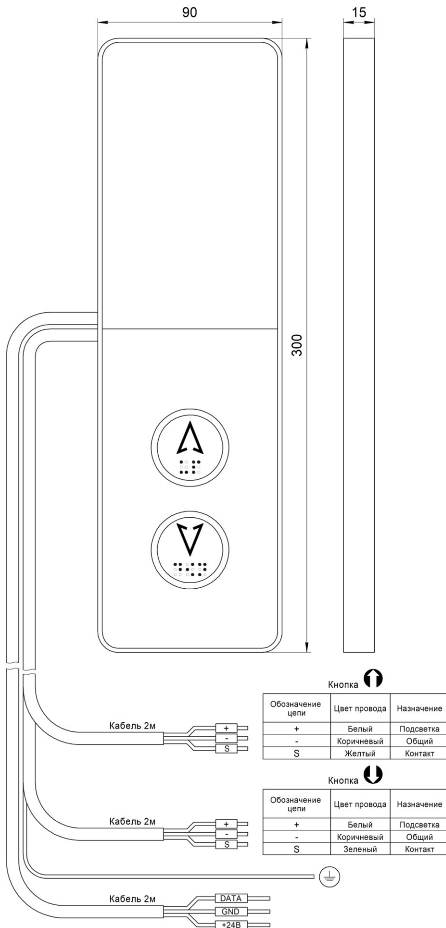
Рис.1 Внешний вид Вызывной пост ОНИКС НШЕК.468381.028
